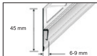
Přechodový profil
