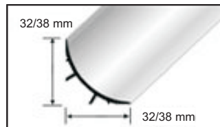
Obloukový profil
