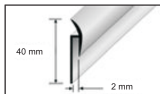
Ukončovací profil
